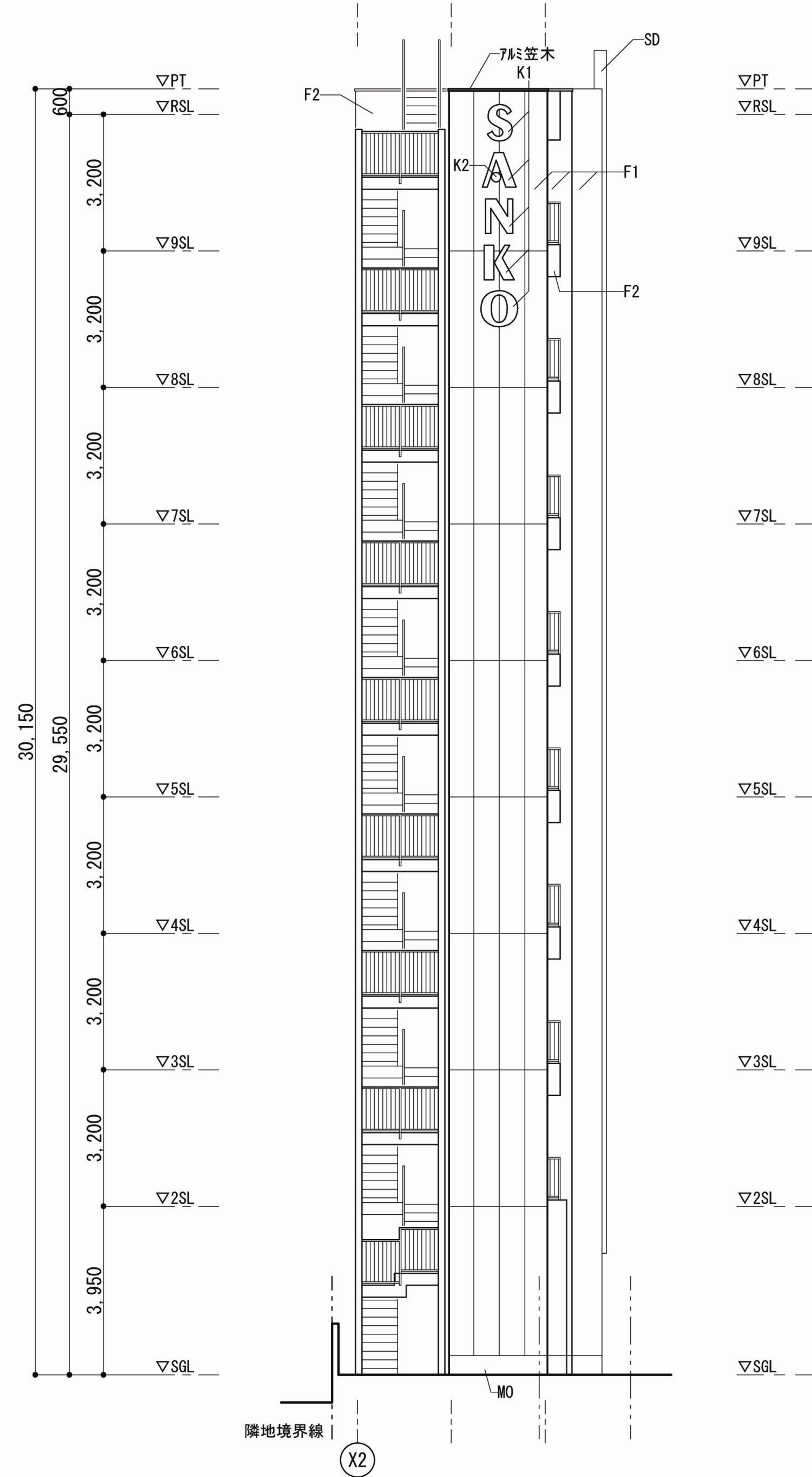
北立面図
