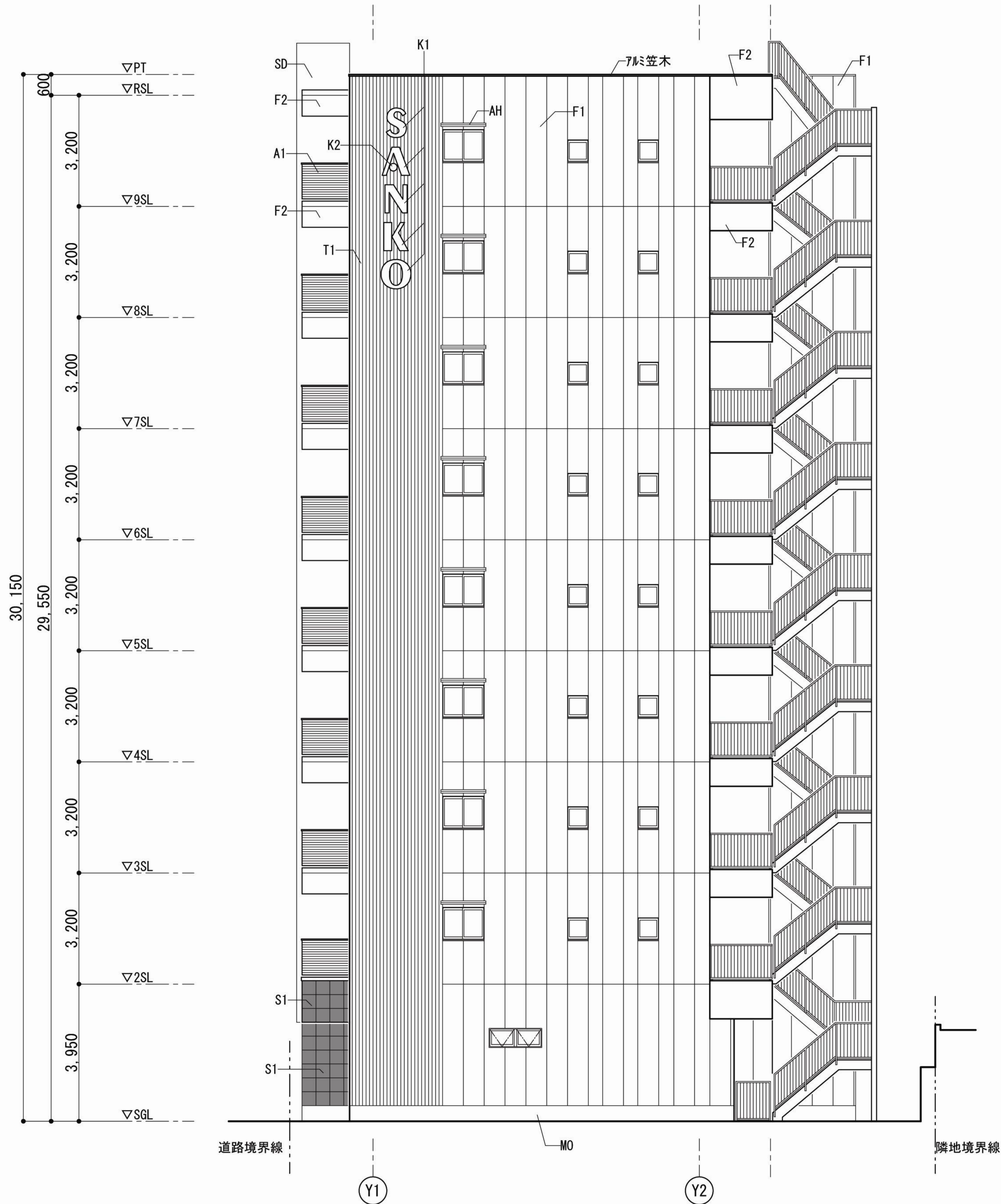
東立面図
