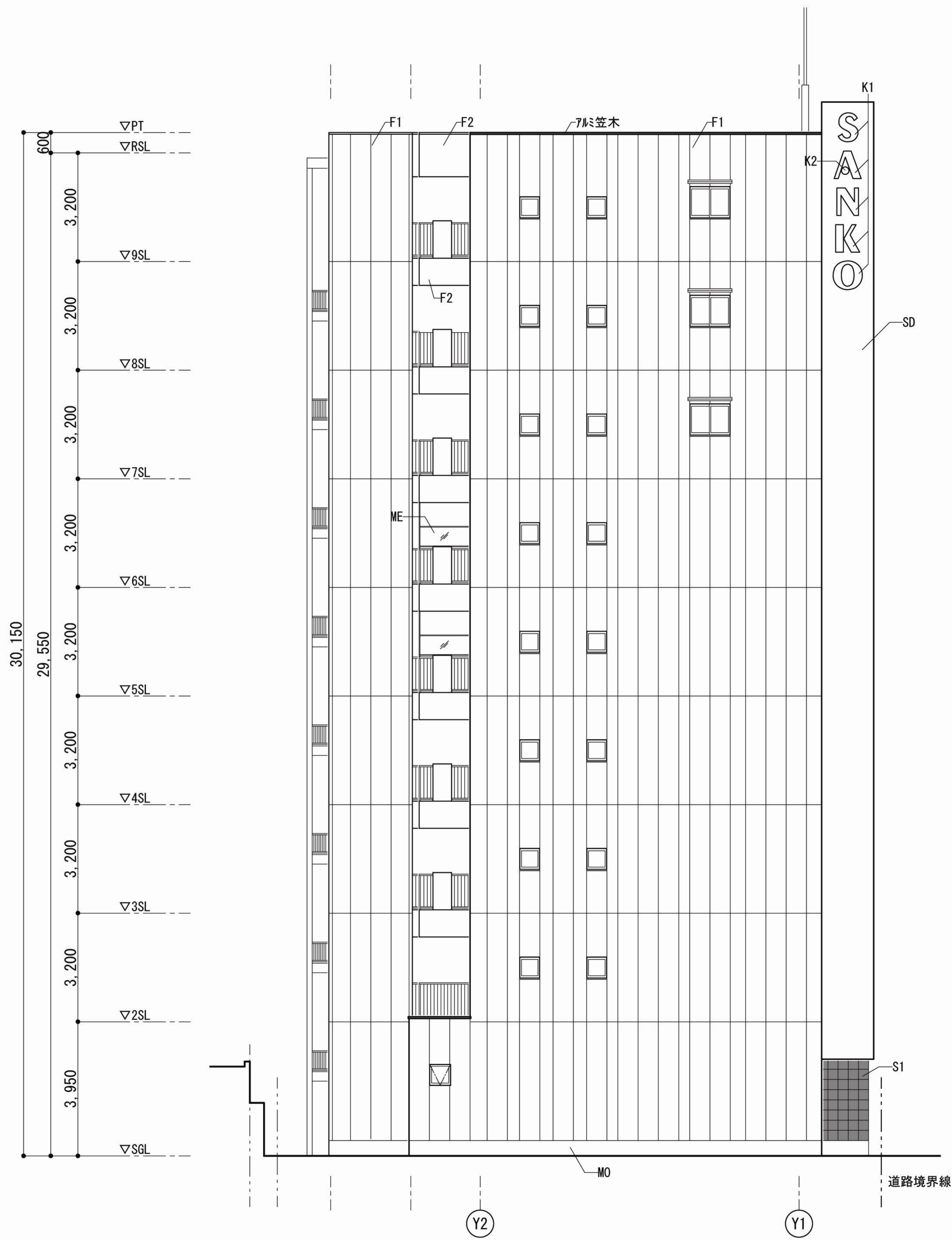
西立面図
